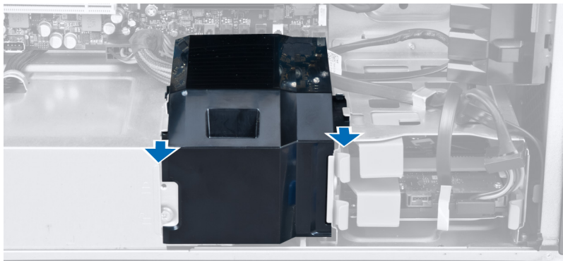
4. Extracción del deflector de la cubierta del equipo.
