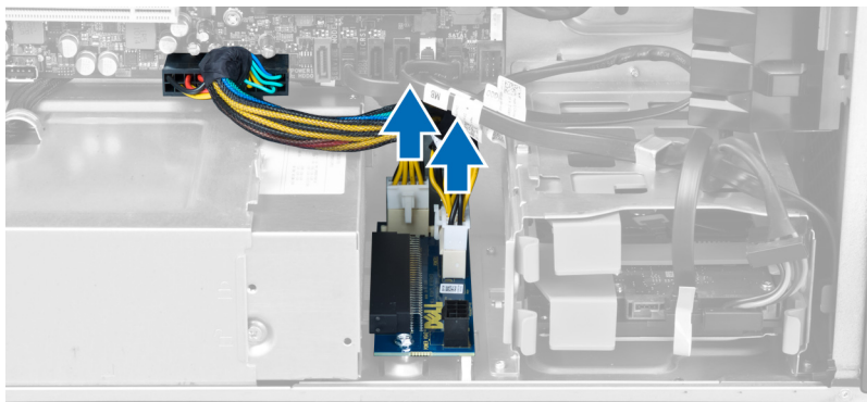
6. Extraiga los tornillos que fijan la tarjeta PSU a su ranura.
